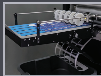
Sistema Transportador con Separador de Sobrantes
